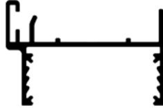
Başlangıç Profili
