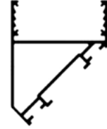
45° Köşe Dönüş Profili
