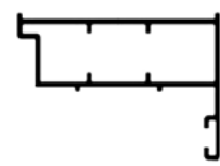
Dikme Profili
